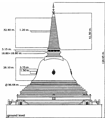
佛统大塔结构图
